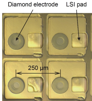
図2 LSI上にダイヤモンド電極を有する集積化バイオセンサーアレイ
